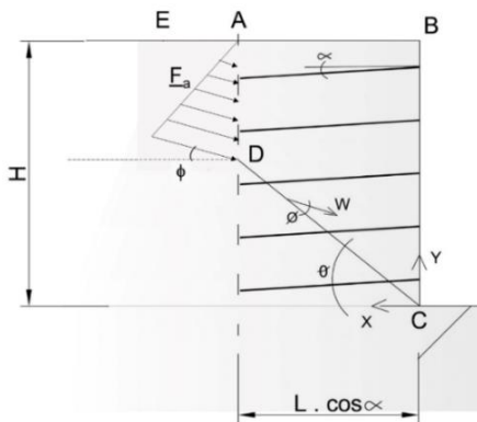
Figure 7. Mécanisme 2 blocs
