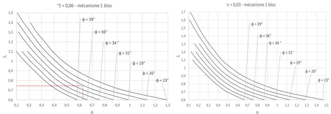
Figure 6. Diagrammes de stabilité pour un mécanisme monobloc – \bar{c} = 6 \% et 3 \%
