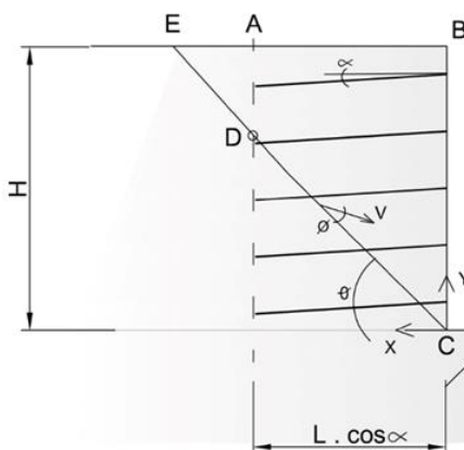
Figure 4. Mécanisme translationnel monobloc
