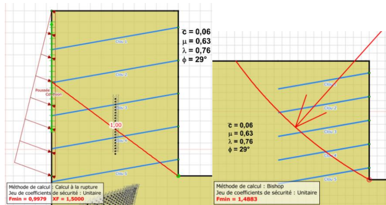
Figure 8. Résultats des calculs Talren
