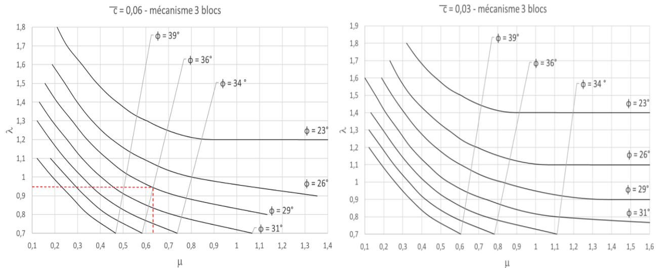
Figure 13. Diagrammes de stabilité pour un mécanisme 3 blocs – \bar{c} = 6 \% et 3 \%
