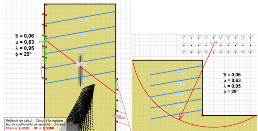
Figure 12. Résultats du calcul Talren
