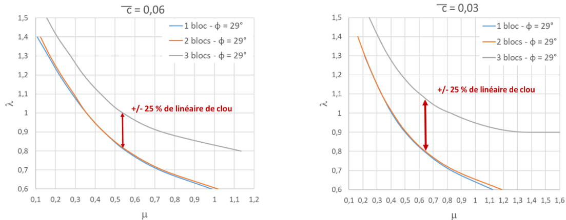
Figure 14. Comparaison des diagrammes de stabilité pour les mécanismes 2 et 3 blocs pour \bar{c} = 6 \% et 3 \% et \phi = 29^\circ
