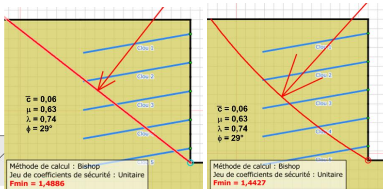
Figure 5. Résultat des calculs Talren
