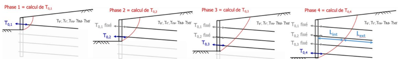
Figure 1. Principe de calcul phasé de la contribution du parement (sans redistribution des efforts)
