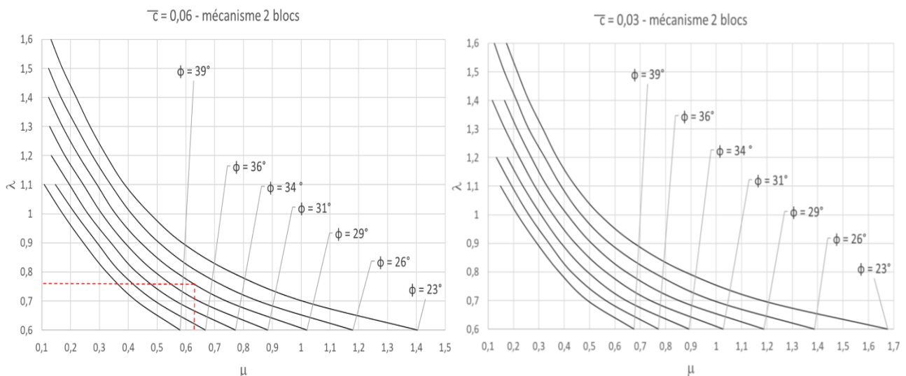
Figure 9. Diagrammes de stabilité pour un mécanisme 2 blocs – \bar{c} = 6\% et 3\%
