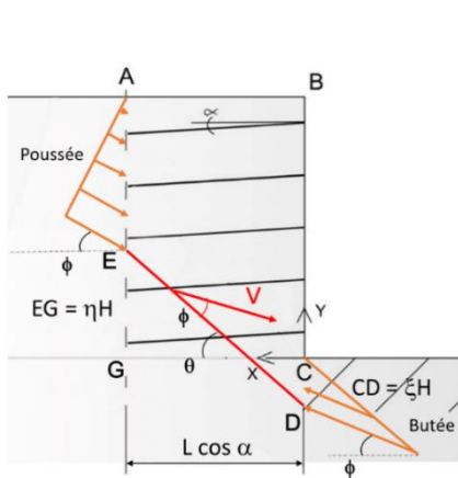
Figure 11. Mécanisme 3 blocs
