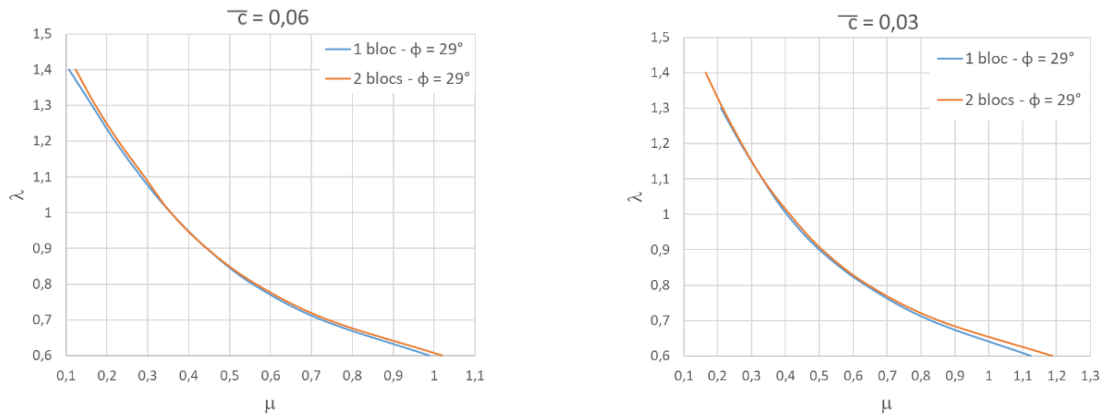
Figure 10. Comparaison des diagrammes de stabilité pour les mécanismes 1 et 2 blocs pour \bar{c} = 6 \% et 3 \% et \phi = 29^\circ
