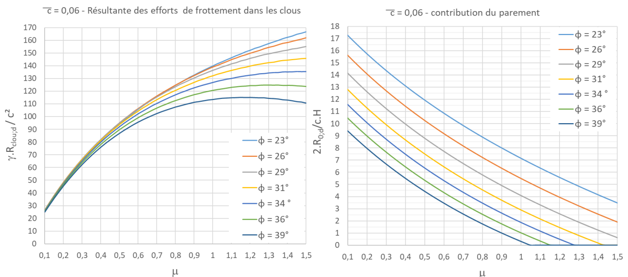
Figure 15. Abaque de prédimensionnement des efforts au parement pour \bar{c} = 6 \%
