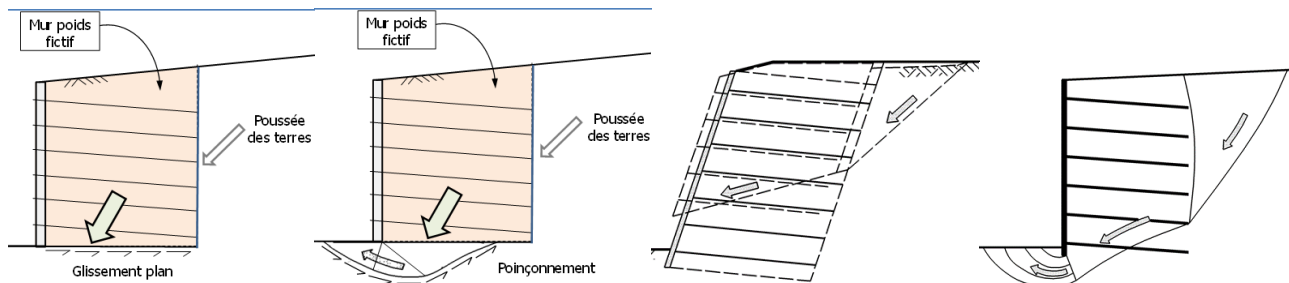
Figure 2. Mécanismes d'instabilité externe Figure 3. Mécanismes d'instabilité 2 blocs et 3 blocs
